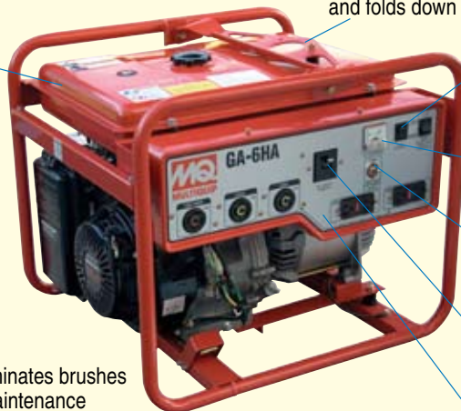
Multiquip GA6HA 6kW Generator
